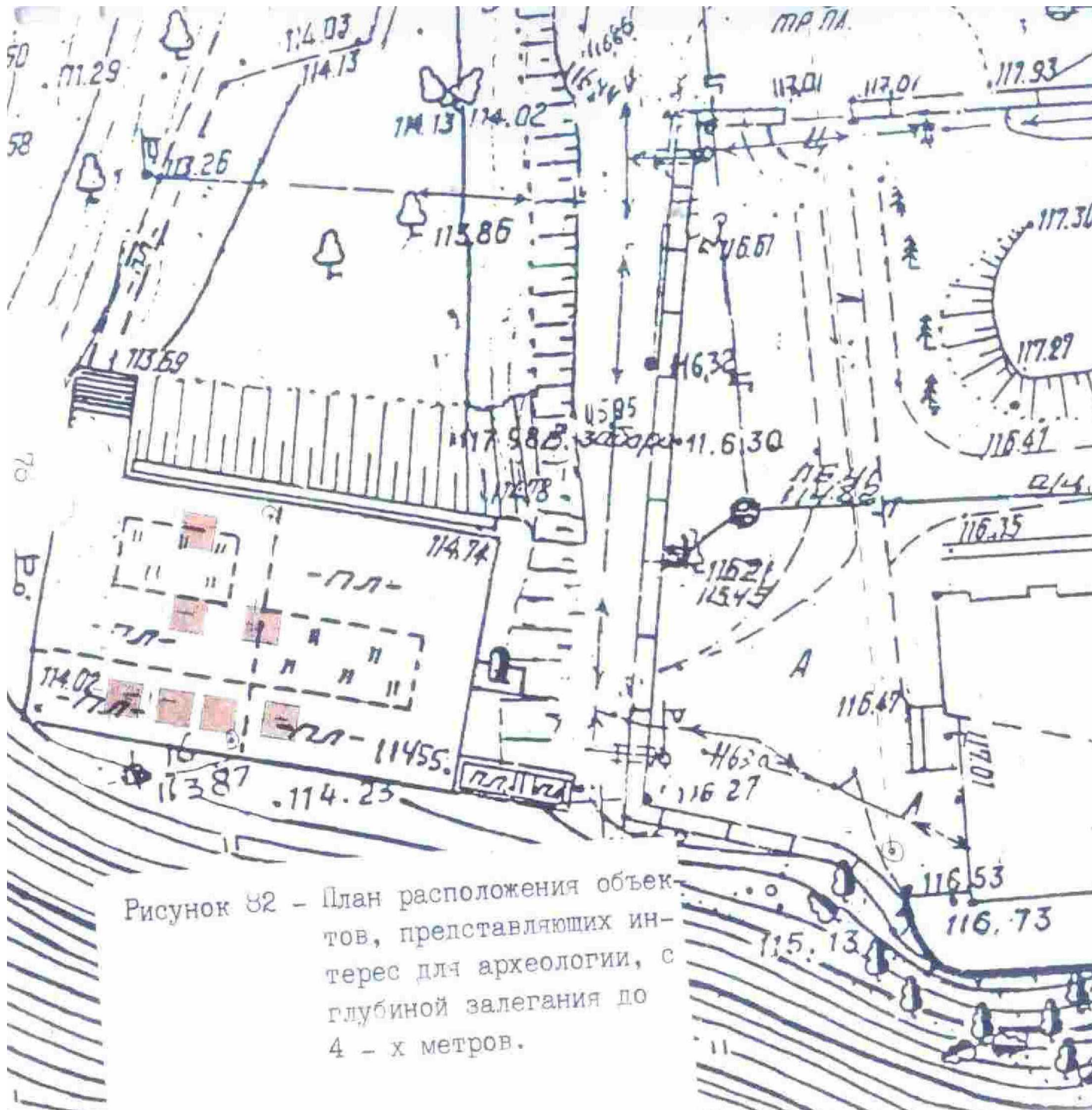
Рис.2 Данные георадара для археологии
